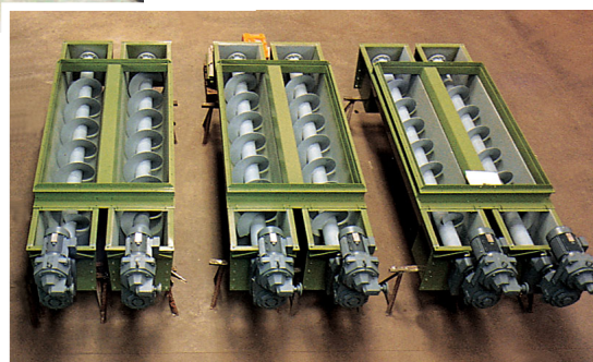
Bunkeraustragung
